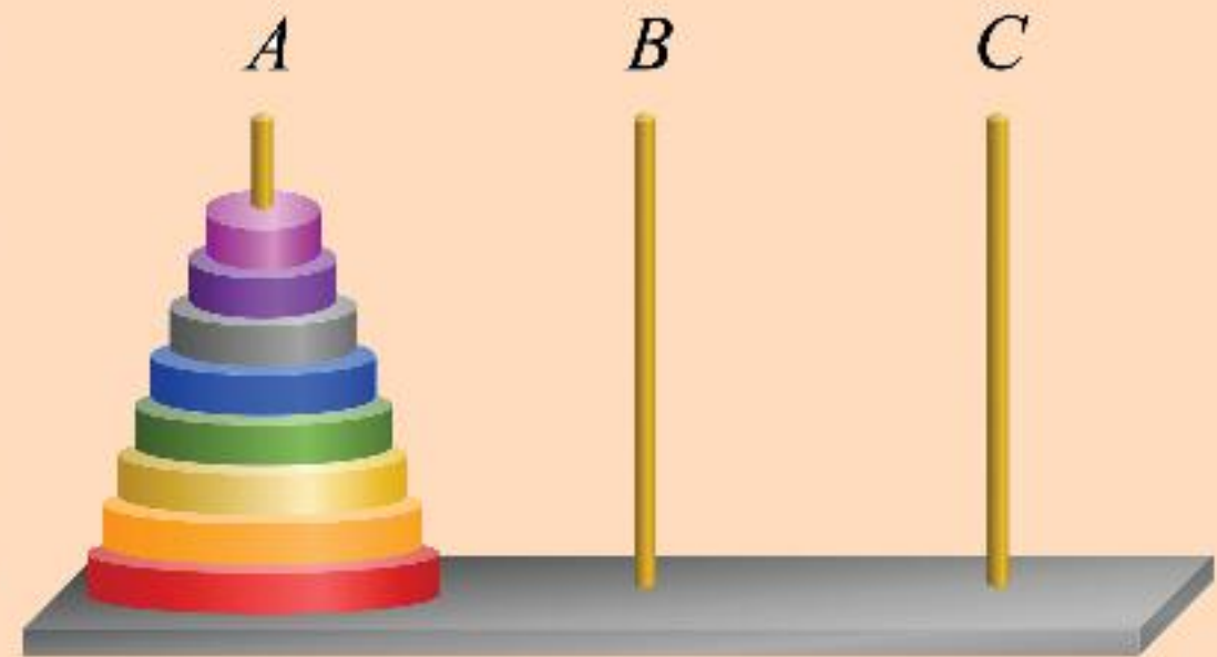
Hình 1. Mô hình Tháp Hà Nội với n = 8
